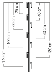
941-035 Montagelehre für Mastschelle
